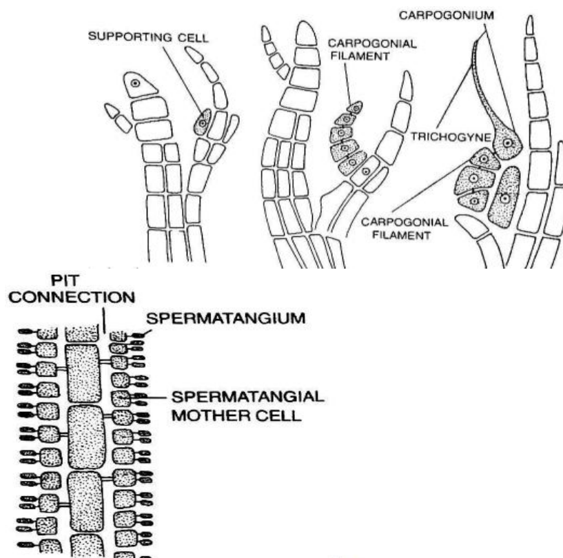
Fig. 3.11 polysiphonia
