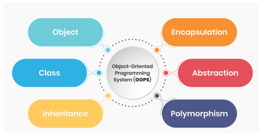
Figure 1.1.1.: OOPs Pillars
