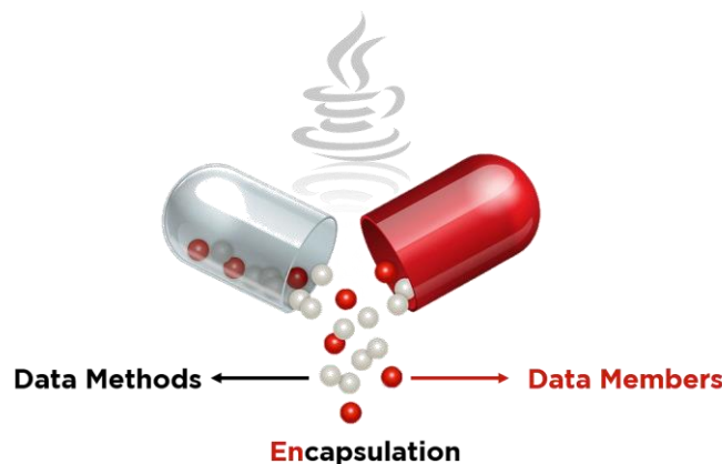
Figure3 : Encapsulation
